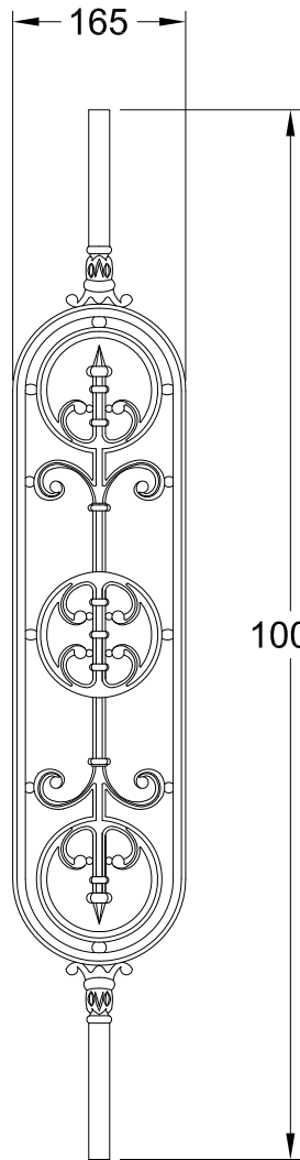
BALUSTER ATDCBA26
